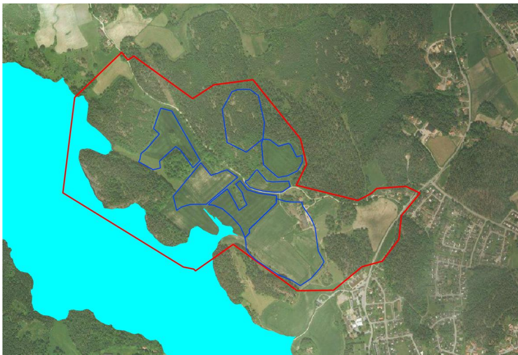
Figur 6. Det turkosa området illustrerar det område som sätts under vatten vid ett 200-årsflöde, dvs en översvämning som statistiskt inträffar 1 gång på 200 år (MSB Portal för översvämningsshot, 2018). Rödmarkering illustrerar planprogramområdesgräns samt de blåmarkerade områdena visar vart bostadsbebyggelsen är tänkt att placeras.
