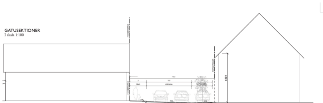
Figur 36. Typsektion för en relativt smal gata, men med längsgående parkering mellan planterade träd.
