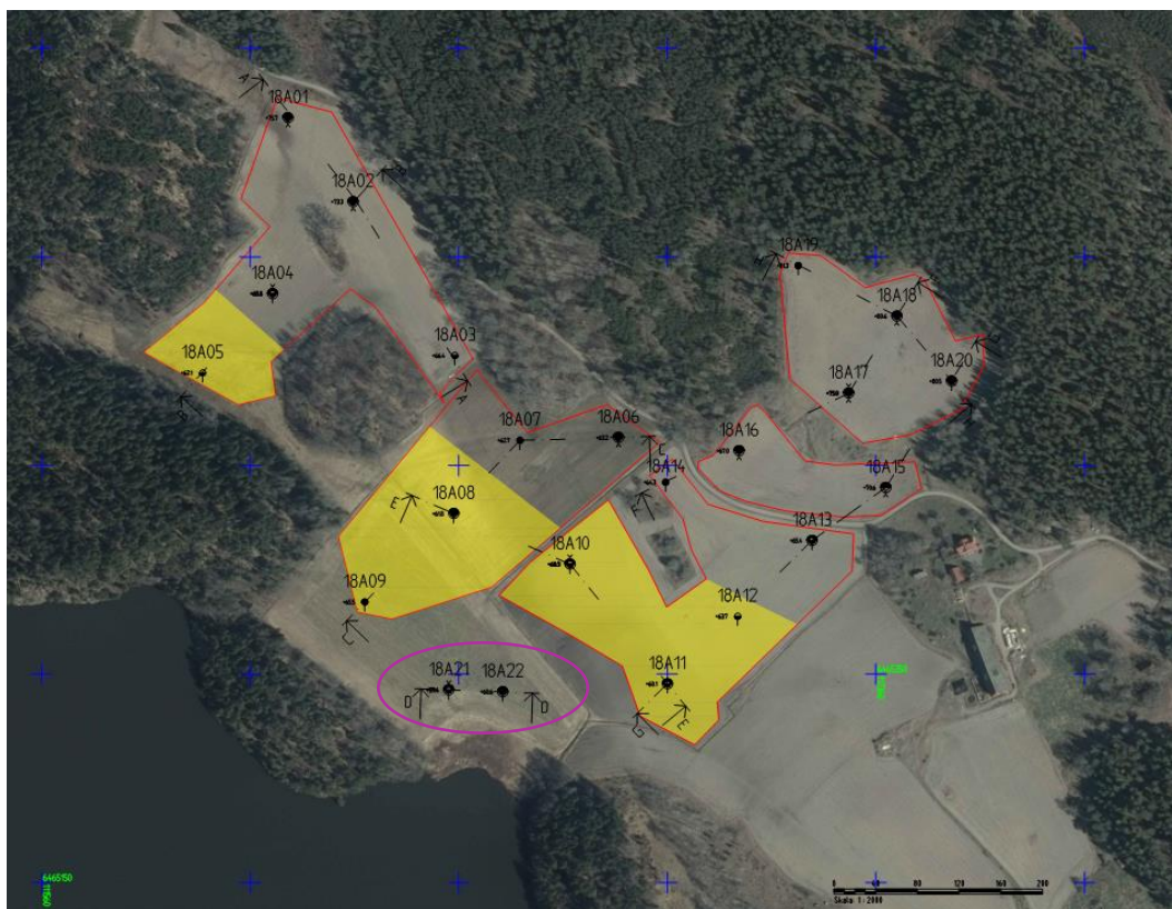
Figur 13. De gulamarkerade områdena representerar delområden, inom områden för planerad bostadsbebyggelse, där det eventuellt kan finnas risk för utveckling av långtidssättningar.
