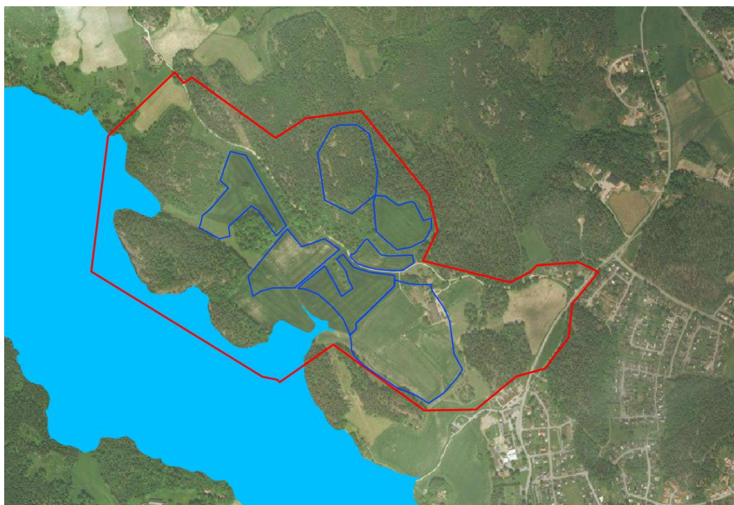
Figur 5. Det blå området illustrerar det område som sätts under vatten vid ett 100-årsflöde, dvs en översvämning som statistiskt inträffar 1 gång på 100 år (MSB Portal för översvämningshot, 2018). Rödmarkering illustrerar planprogramområdesgräns samt de blåmarkerade områdena visar vart bostadsbebyggelsen är tänkt att placeras.
