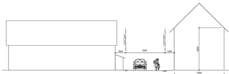
Figur 33. Typsektion för det mindre gaturummet som ger en mer intim känsla och fungerar som gårdsgator där trafiken sker på fotgängarnas villkor.
