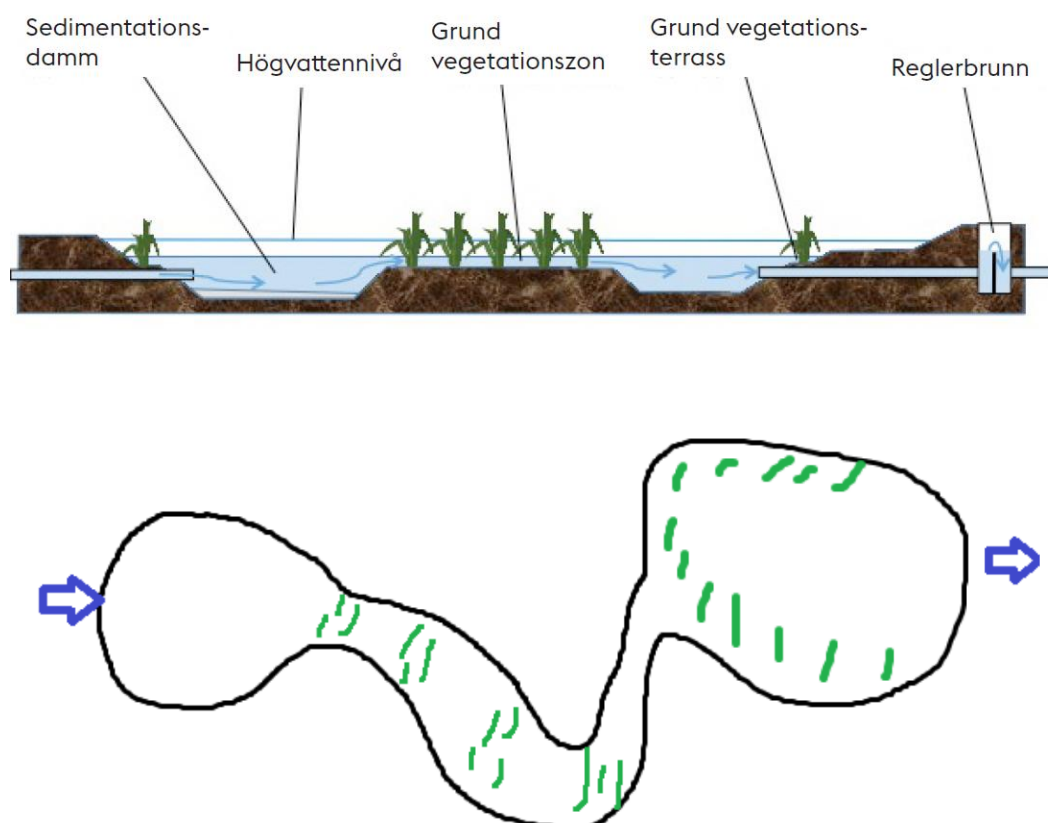
Figur 21. Principskisser dagvattendamm. (Illustration: Stockholm Stad samt Uppsala Vatten).
